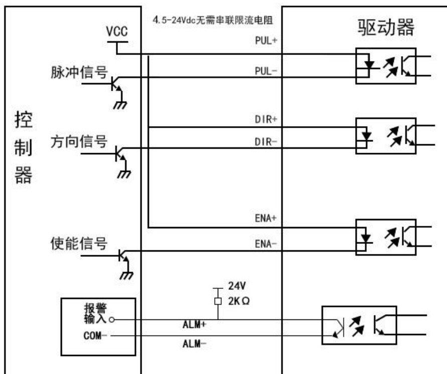
共阳极接法
