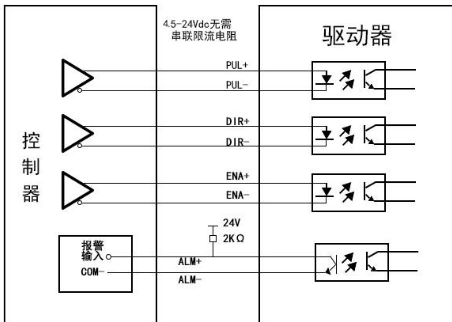
差分方式控制信号接口接线图
