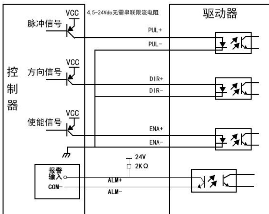
共阴极接法
