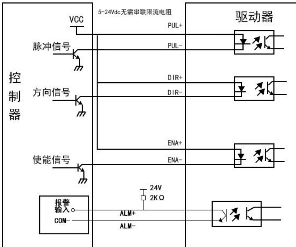
共阳极接法
